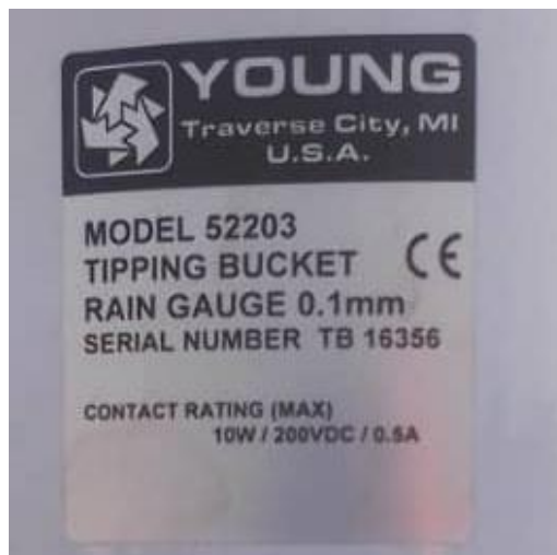
Figure 26: Numéro de série du capteur de pluie / Rain sensor serial number
