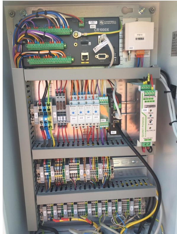
Figure 94: Intérieur de l'armoire principale / Interior of main cabinet.
