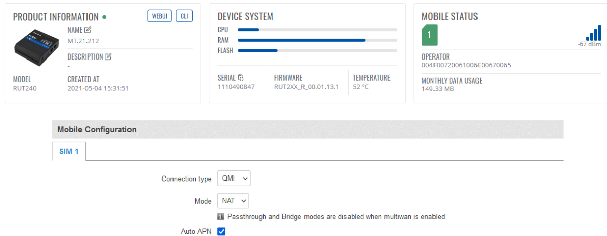
Figure 11: État de communication du routeur LTE pour la transmission de données / Communication status of LTE router for data transmission.
