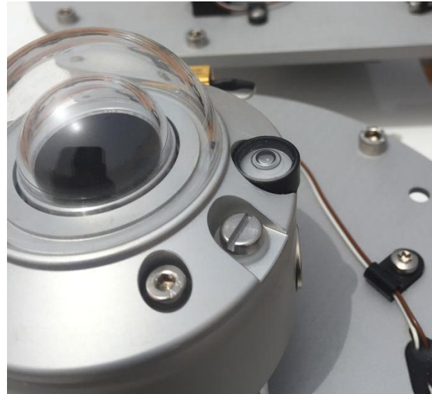
Figure 53: Mise à niveau du pyranomètre CMP10 (GHI) / CMP10 pyranometer leveling (GHI).
