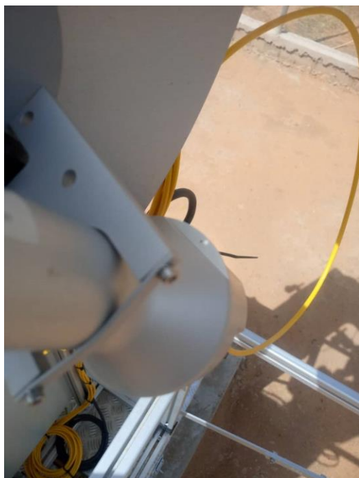
Figure 93: Alignement du pyrhéliomètre avant correction / Pyrheliometer alignment before correction.
