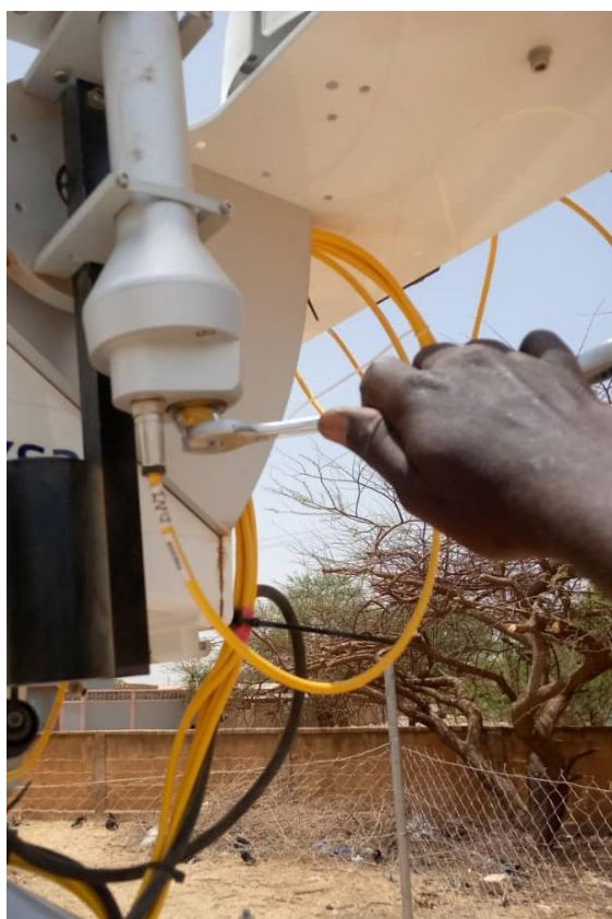
Figure 83 : Changement du disséquant de Pyrliometer / Change of pyrliometer desiccant.
