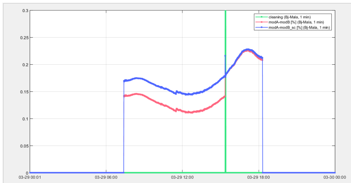
Figure 33: Procédure d'évaluation des salissures du panneau de référence (exemple) / Reference panel soiling assessment procedure (exemple).
