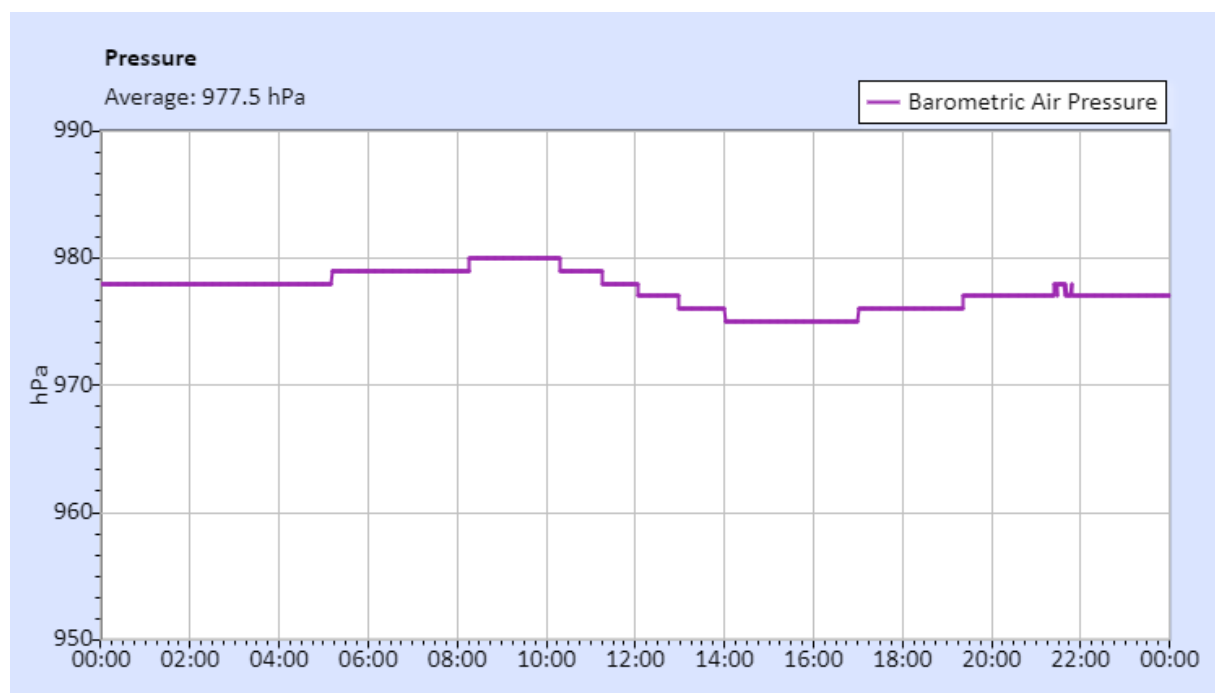
Figure 15 : Mesure de la pression atmosphérique barométrique / Barometric air pressure measurement.
