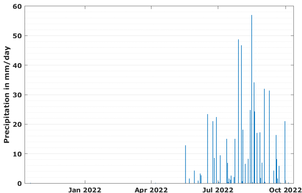
Figure 27: Sommes journalières des précipitations / Daily sums of precipitation.
