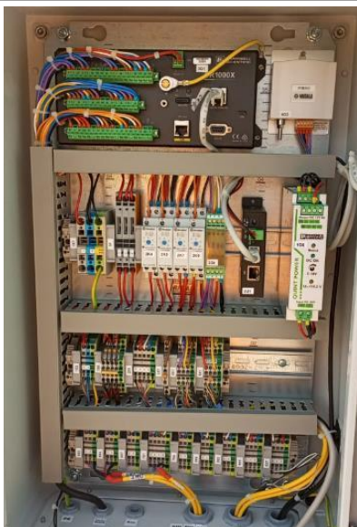
Figure 65: Intérieur du boîtier de contrôle / Control box interior.
