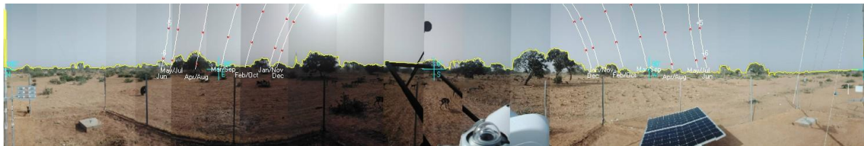
Figure 3: Ligne d'horizon du point de vue du pyranomètre et course du soleil tout au long de l'année / Horizon line from the perspective of the pyranometer and sun path throughout the year.
