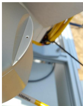
Figure 28 : Alignement du pyrhéliomètre / Pyrheliometer alignment
