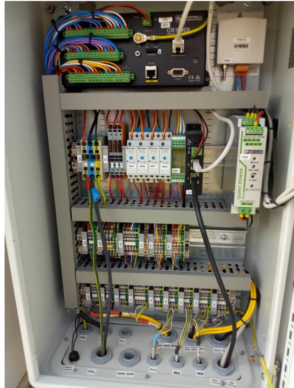
Figure 89 : Intérieur de l'armoire principale / Interior of main cabinet.
