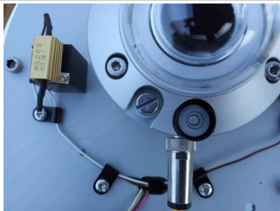
Figure 53: Mise à niveau du pyranomètre CMP10 (GHI) / CMP10 pyranometer leveling (GHI).
