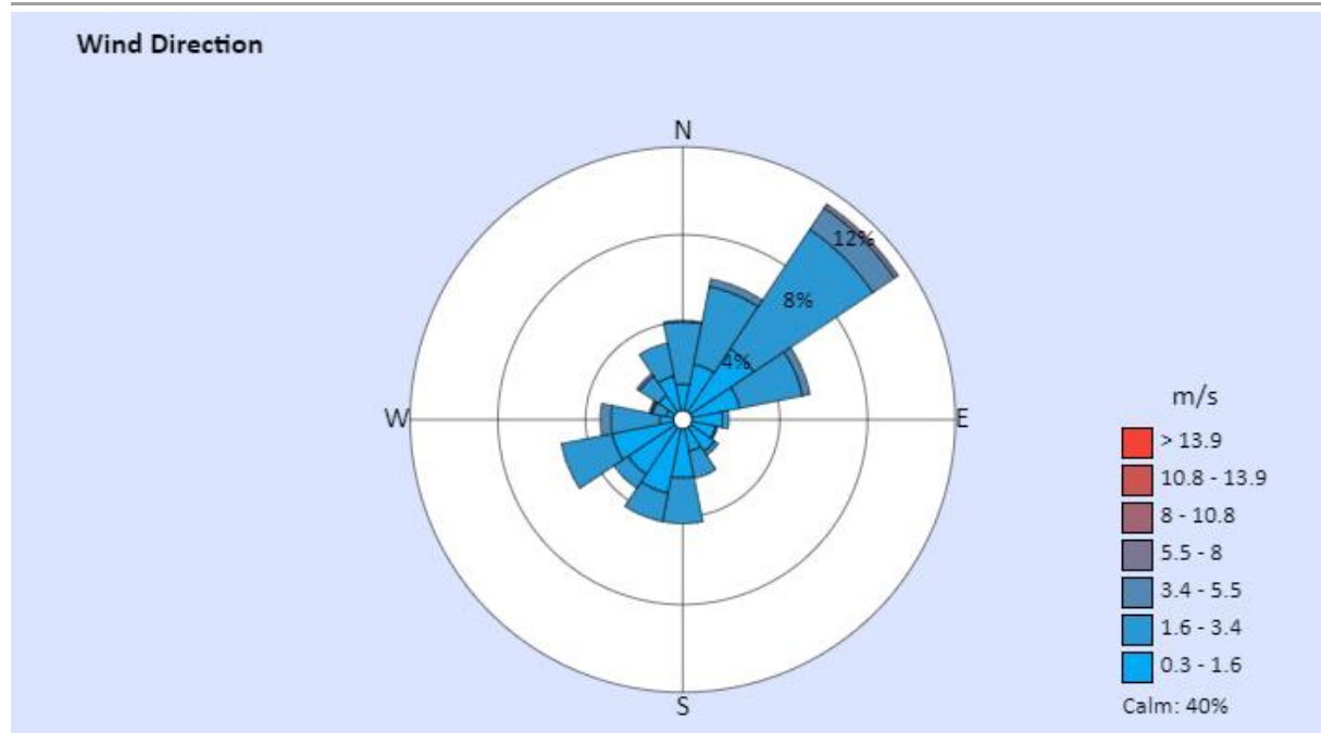
Figure 18 : Mesure direction du vent / Wind direction measurement.
