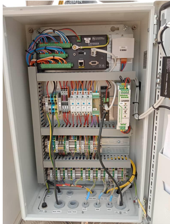
Figure 93 : Intérieur de l'armoire principale / Interior of main cabinet.
