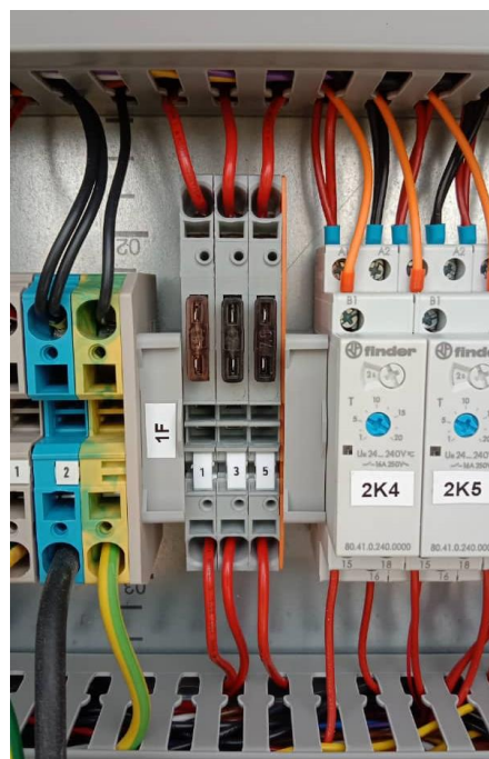
Figure 79: Alimentation électrique de la station rétablie / Restored station power supply.
