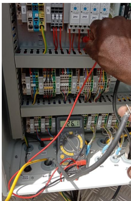
Figure 99: Alimentation électrique reconnectée / Power supply reconnected.
