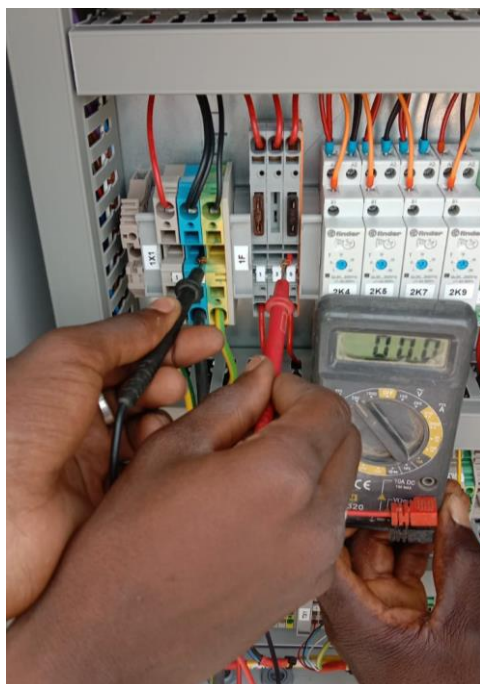
Figure 76: Mesures de la tension de l'alimentation électrique / Power supply voltage measurements.
