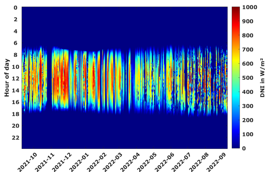
Figure 24: : Intensité de la DNI / DNI irradiance intensity.
