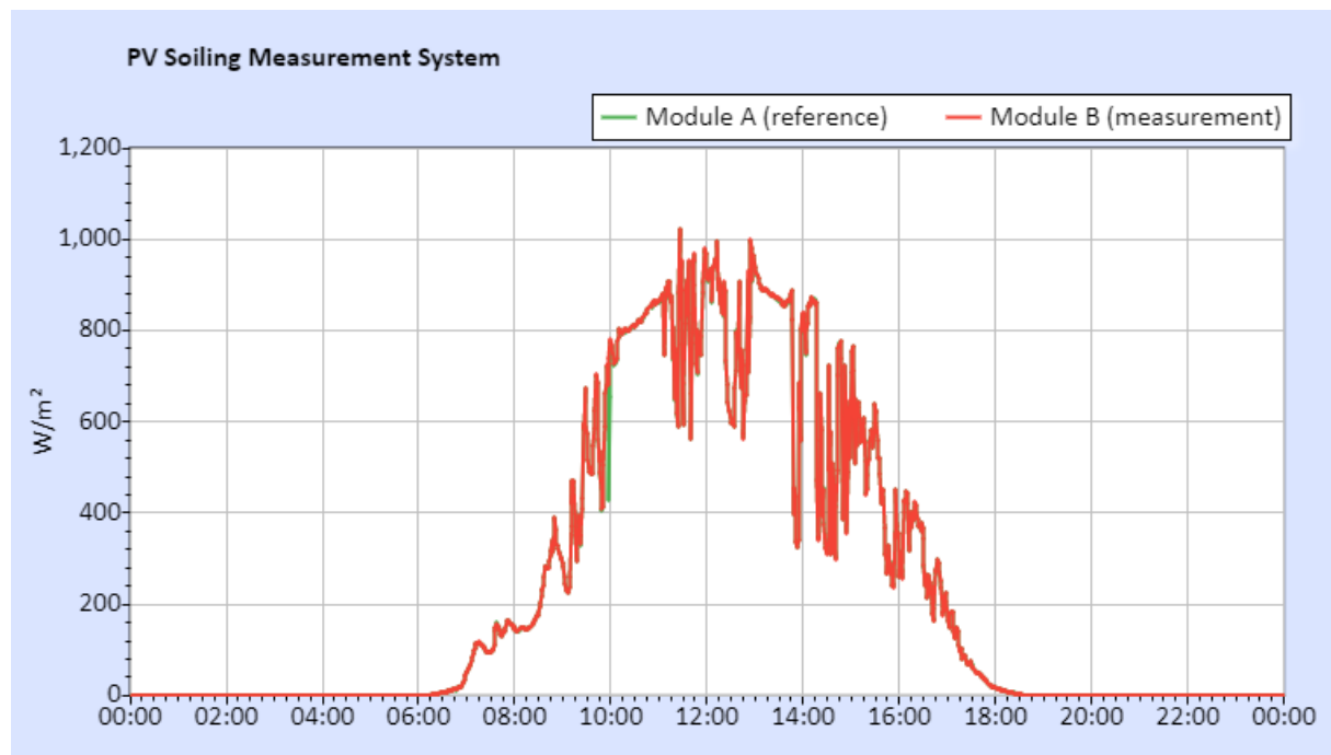
Figure 19 : PV Mesure d'encrassement des panneaux PV / PV soiling measurements.
