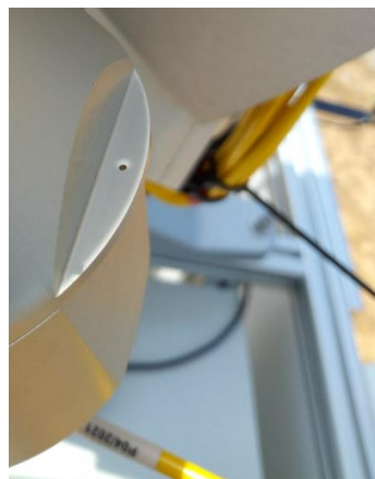
Figure 63 : Alignement du pyrhéliomètre / Pyrheliometer alignment.
