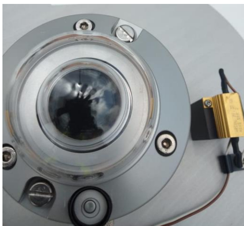
Figure 19: Mise à niveau du pyranomètre CMP10 (GHI) / CMP10 pyranometer leveling (DHI)
