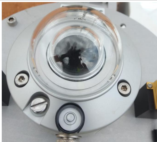
Figure 18: Mise à niveau du pyranomètre CMP10 (GHI) / CMP10 pyranometer leveling (GHI)
