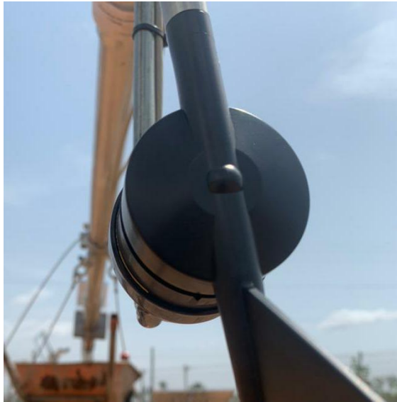
Figure 48: Marque nord du capteur de direction du vent alignée avec le cantilever de montage et la direction du nord. / Wind direction sensor north mark aligned with mounting cantilever and north direction.
