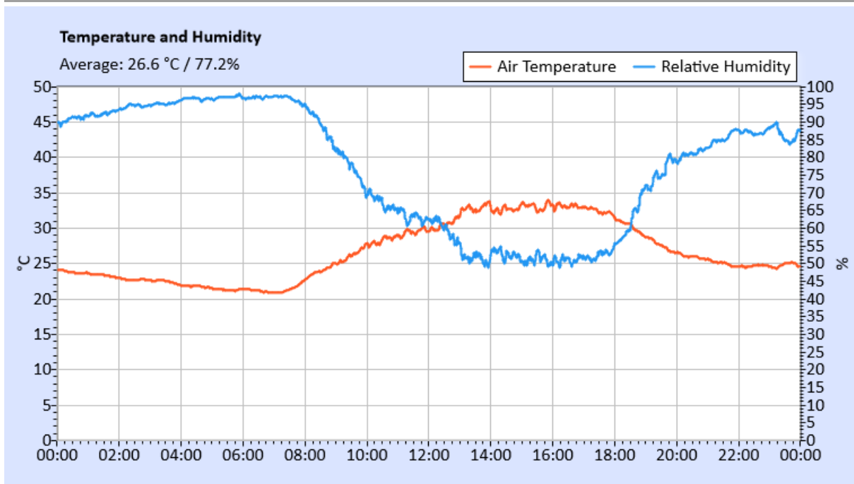
Figure 14: Mesures de la température et de l'humidité / Temperature and Humidity measurements.
