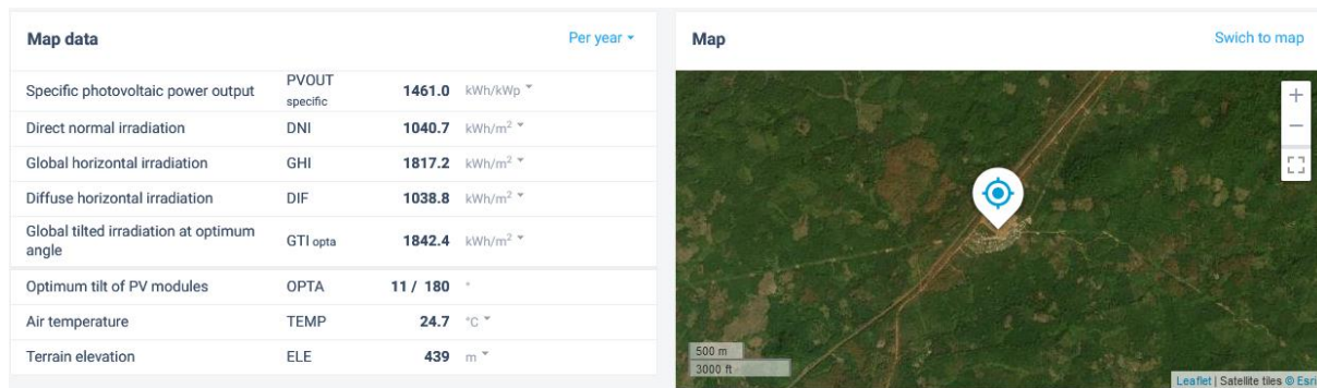
Figure 42: Valeurs moyennes annuelles obtenues à partir du Global Solar Atlas pour le site de Yekepa, Liberia / Yearly average values obtained from the Global Solar Atlas for the site in Yekepa, Liberia.
