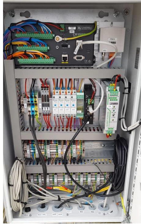
Figure 88 : Intérieur de l'armoire principale / Interior of main cabinet.
