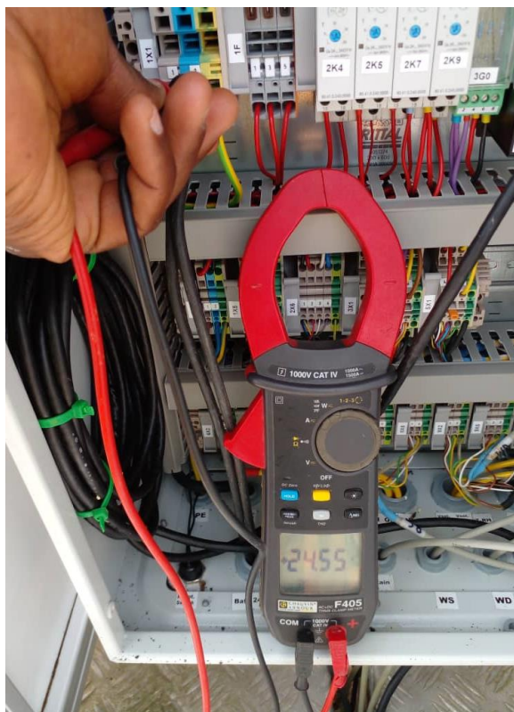
Figure 92: Vérification de la connexion de l'alimentation électrique / Check of power supply connection.
