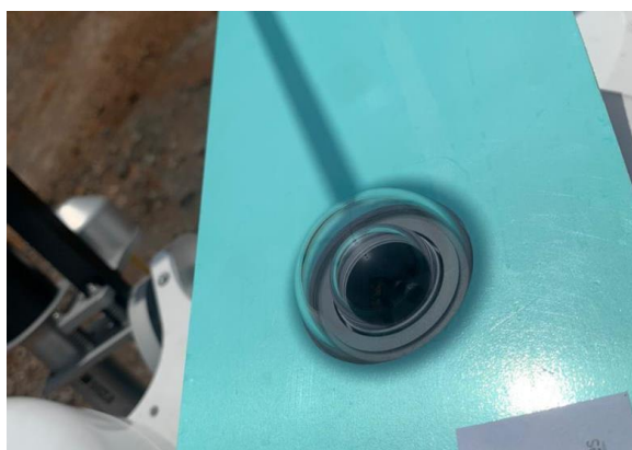
Figure 27: Mise à niveau du dispositif d'ombrage / Shading assembly alignment
