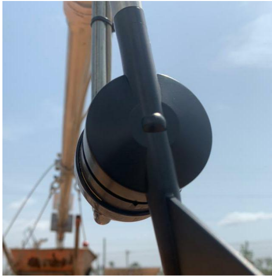
Figure 13: Marque nord du capteur de direction du vent alignée avec le cantilever de montage et la direction du nord. / Wind direction sensor north mark aligned with mounting cantilever and north direction
